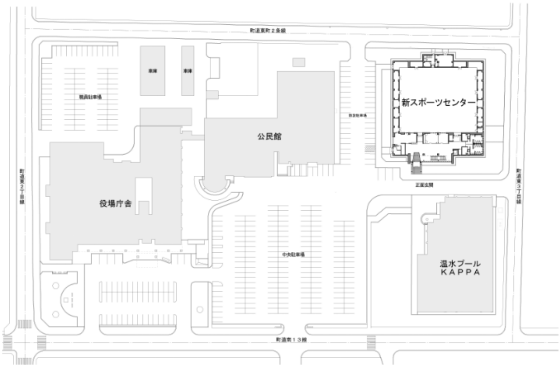
配置図
